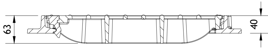
A-A (1:3)
