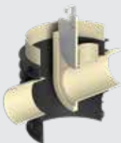
Zwischenteil mit DN/OD 160 Zulauf & Ablauf inkl. Schieber & Überlauf
