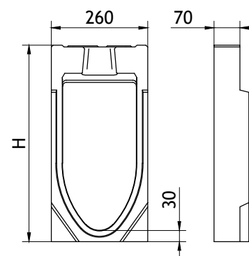
Adapter za bočni priključak
