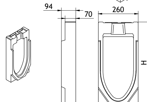
Čeoni poklopac za kraj
