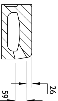
Presek A-A
