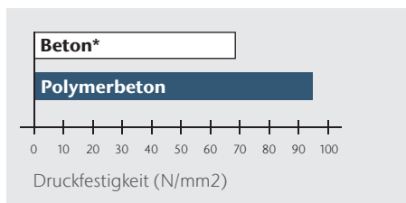
Druckfestigkeiten
